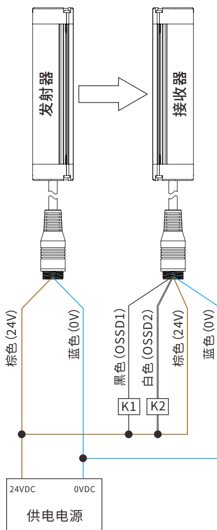
线标说明
