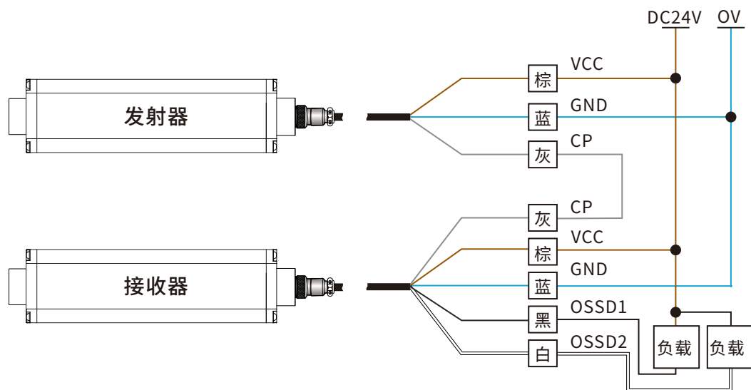
PN接线图
