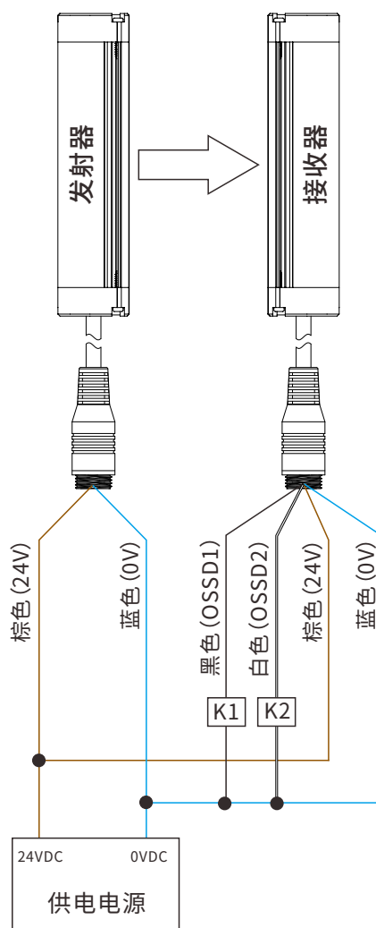
PNP接线图
